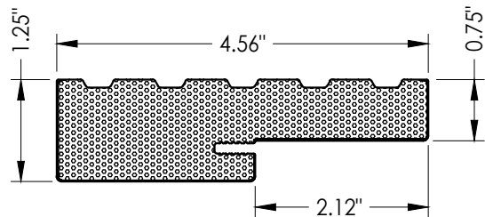
1 JAMB
